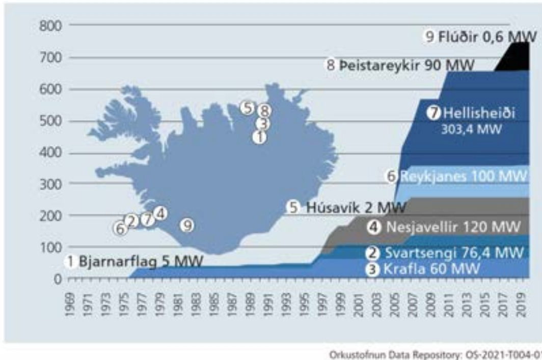
Aineisto 4.9 Geotermisten voimalaitosten sähköteho, sijainti ja toiminta-aika Islannissa.
