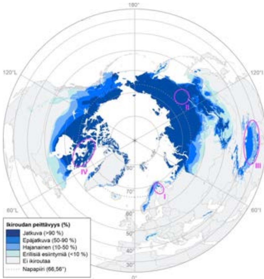
Kuva 3.A. Ikiroudan peittävyys
