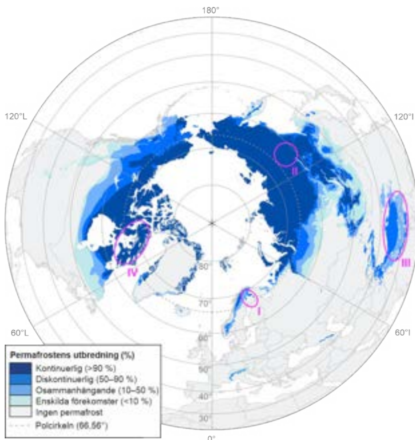
Bild 3.A Permafrostens utbredning
